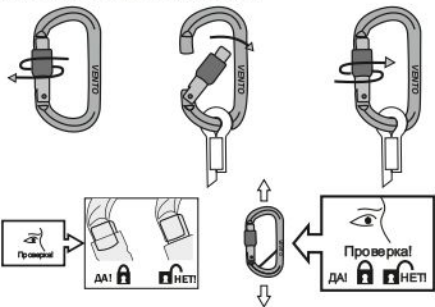
Рис. 3. Использование карабинов
